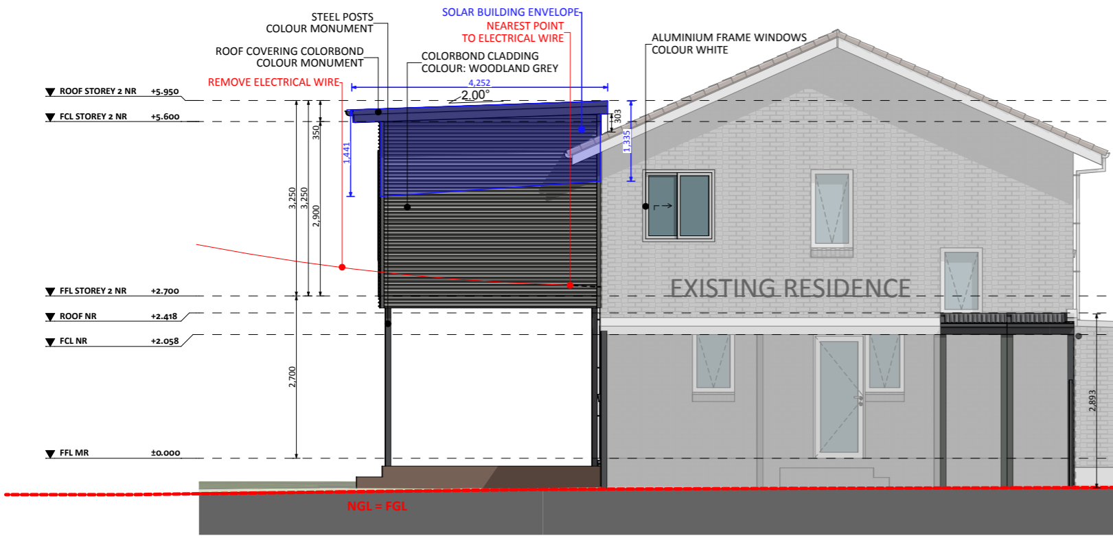
ELEVATION 01
