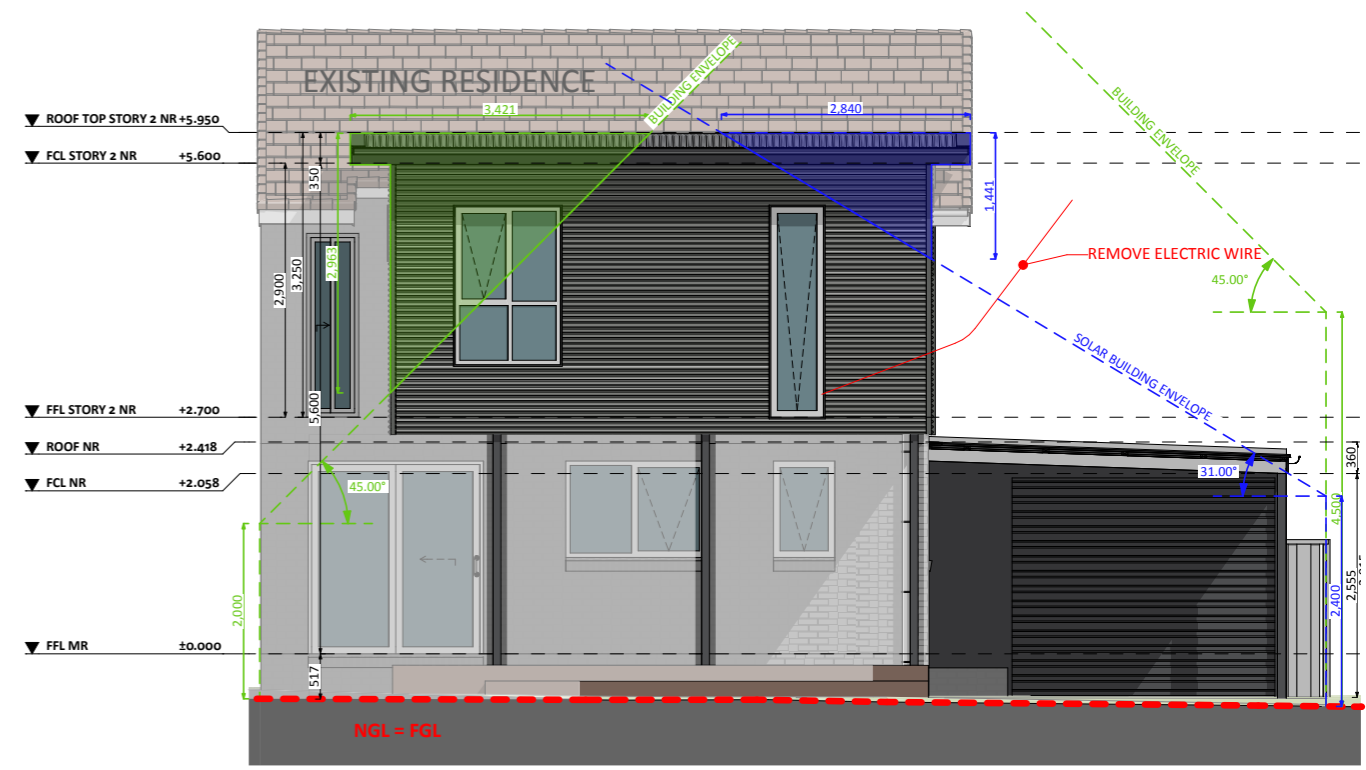
ELEVATION 02
