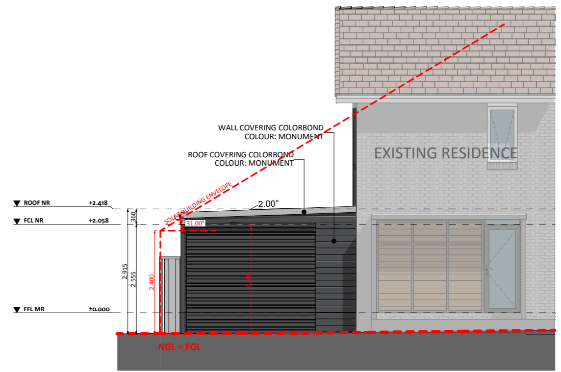
ELEVATION 04
