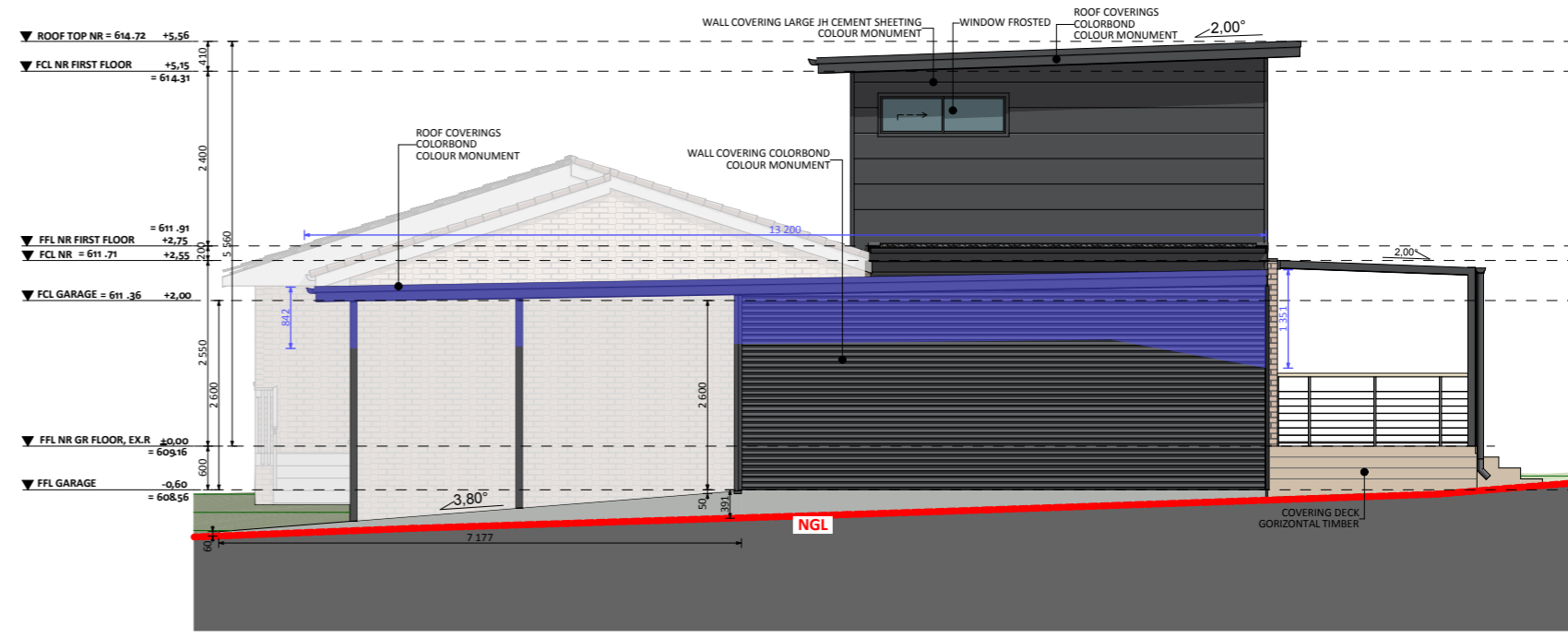
ELEVATION 04
