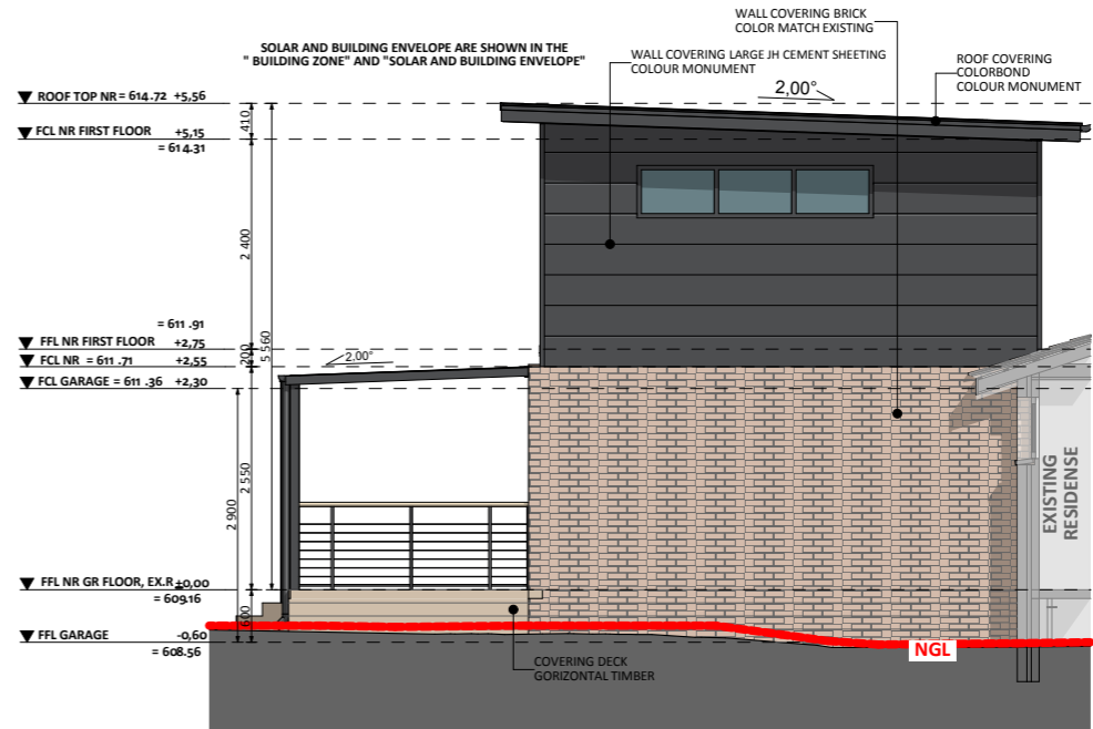
ELEVATION 02
