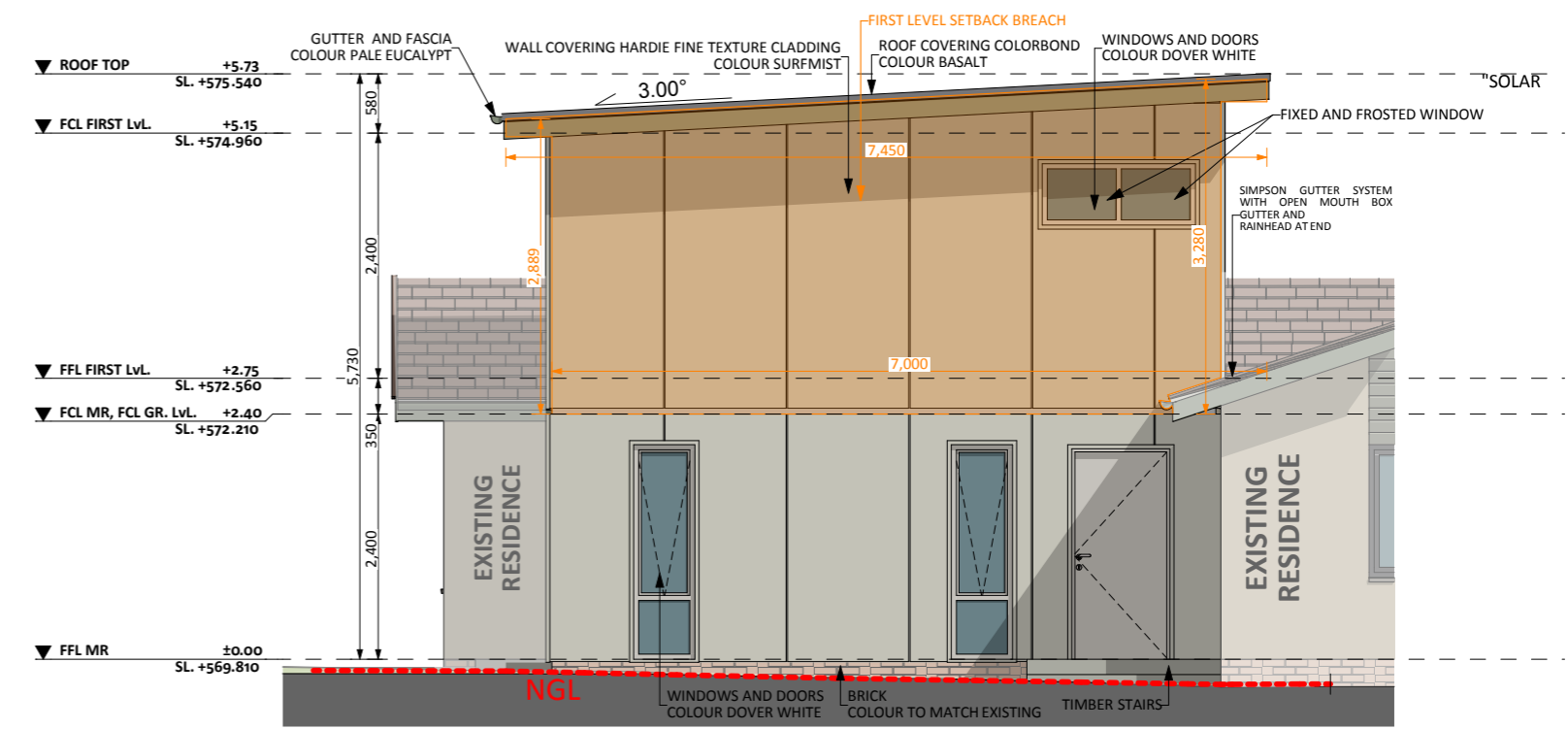
ELEVATION 02
