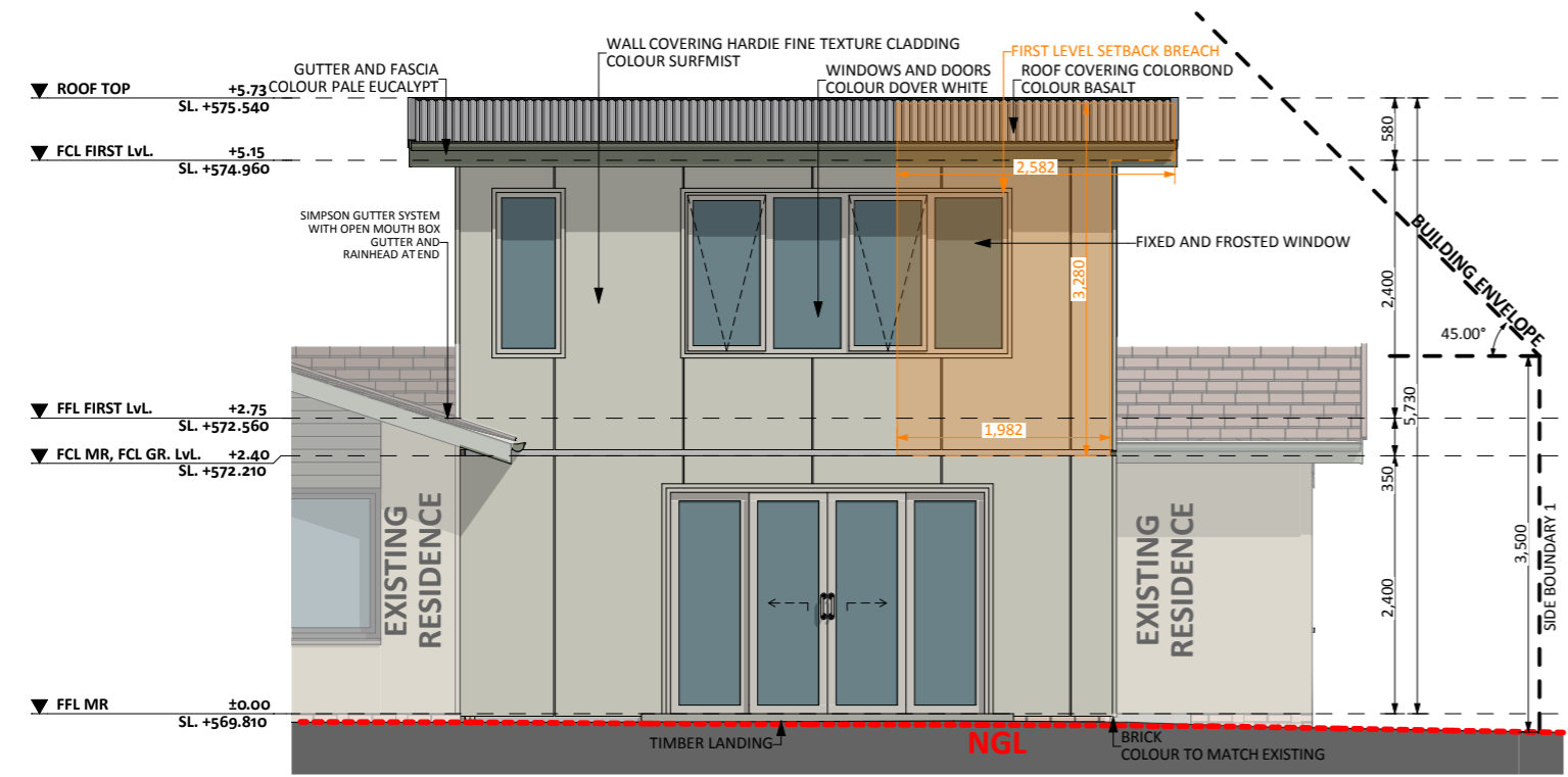
ELEVATION 01
