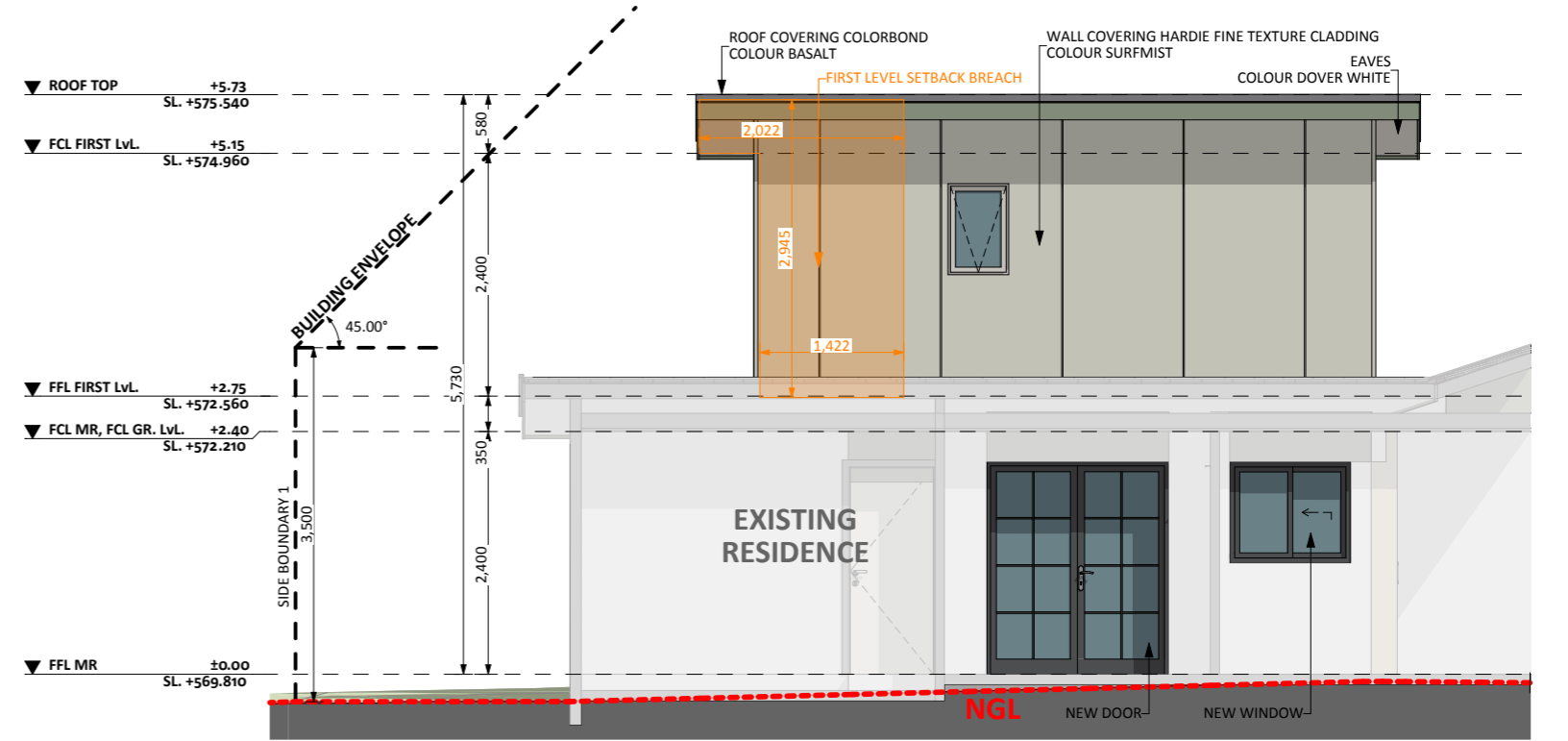
ELEVATION 04
