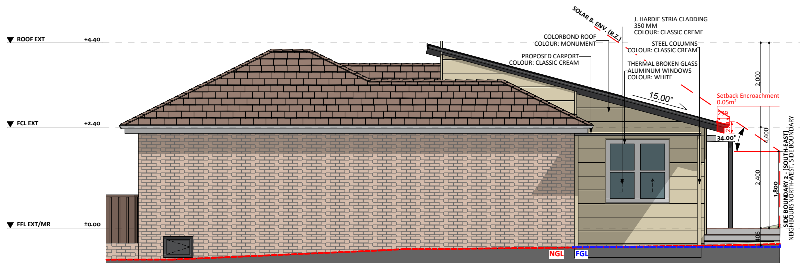
ELEVATION 02
