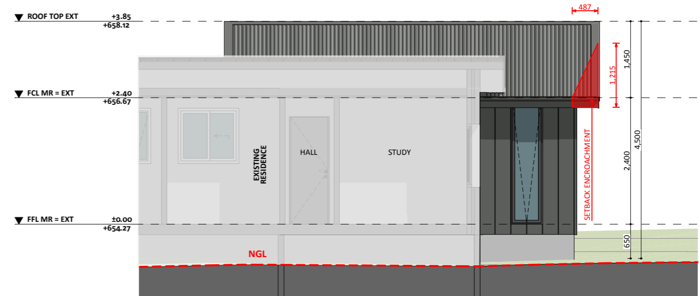
ELEVATION 04
