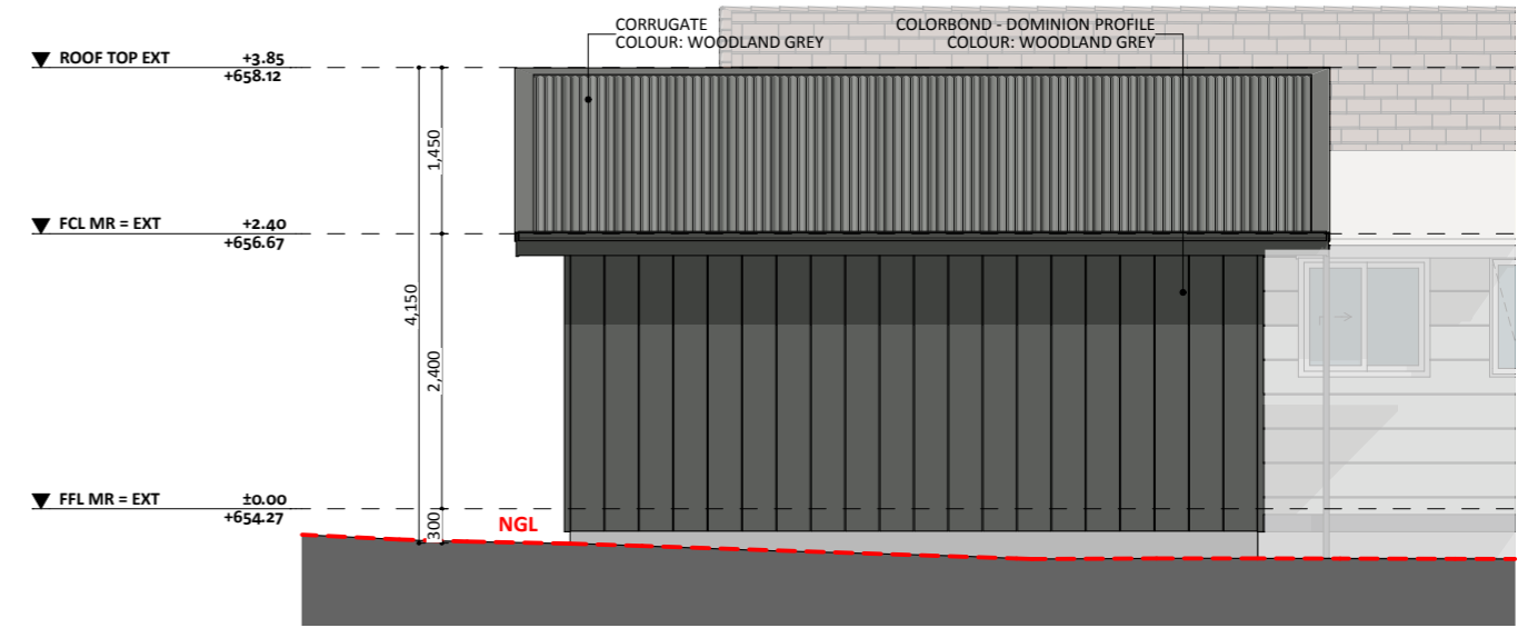
ELEVATION 02
