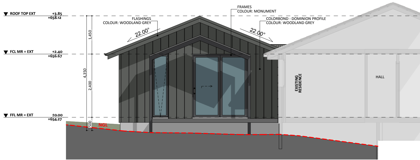
ELEVATION 01
