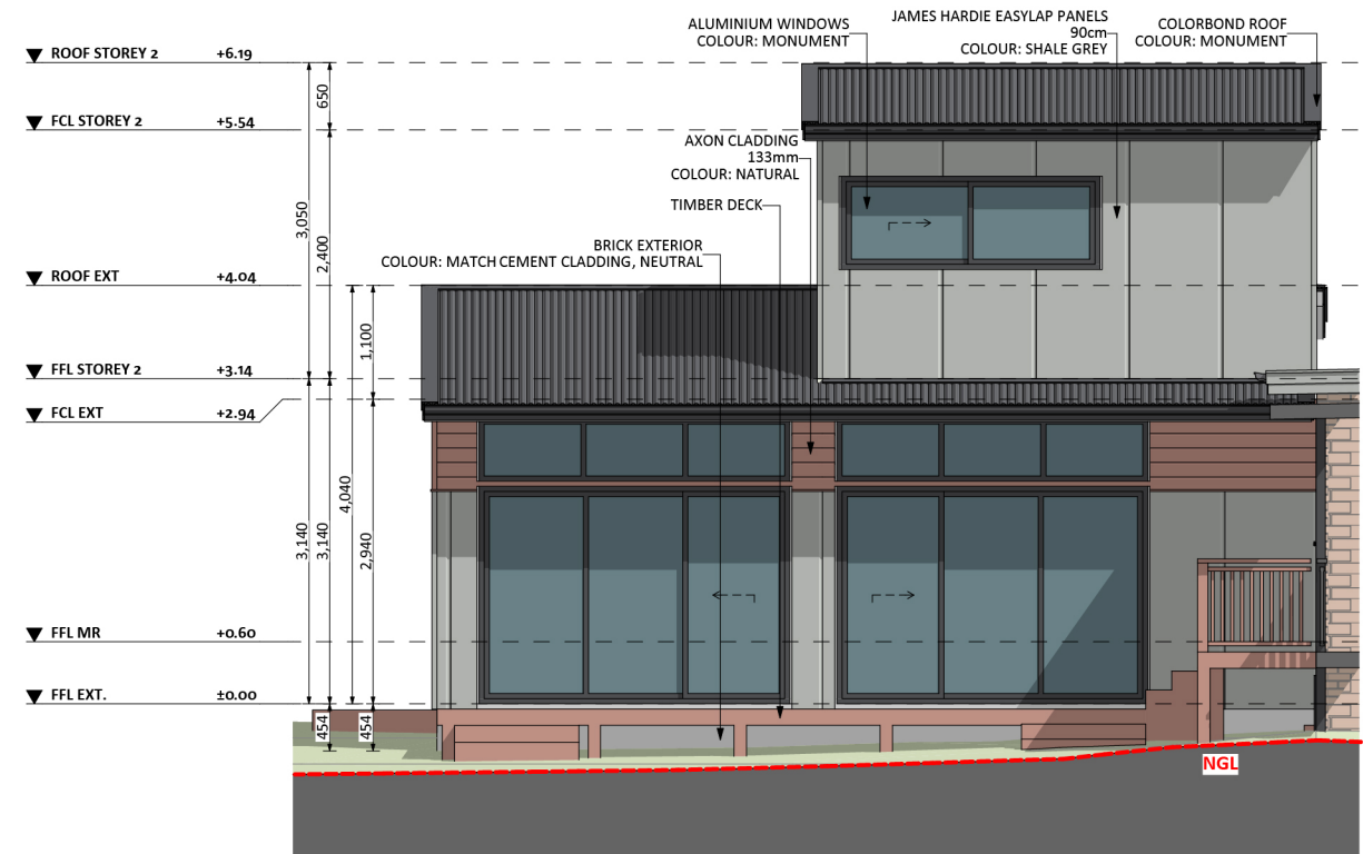
ELEVATION 02
