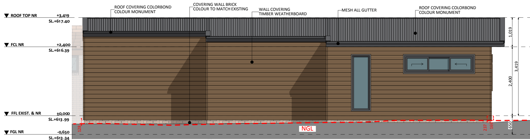
ELEVATION 04
