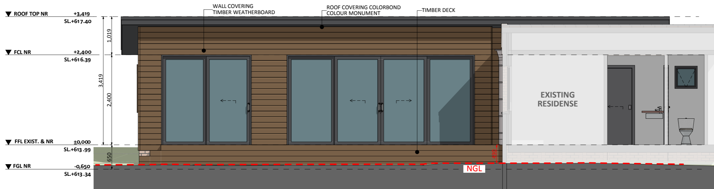
ELEVATION 01
