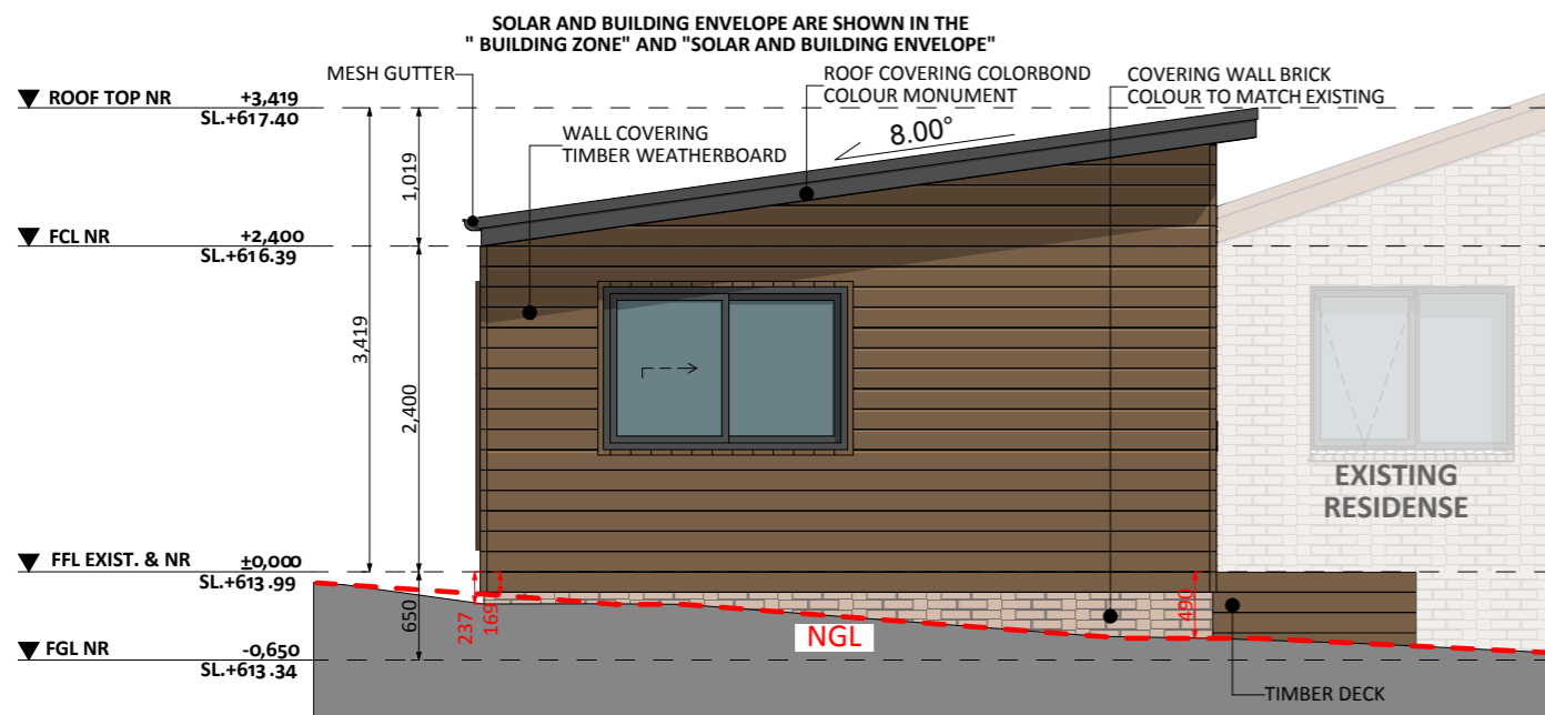
ELEVATION 02
