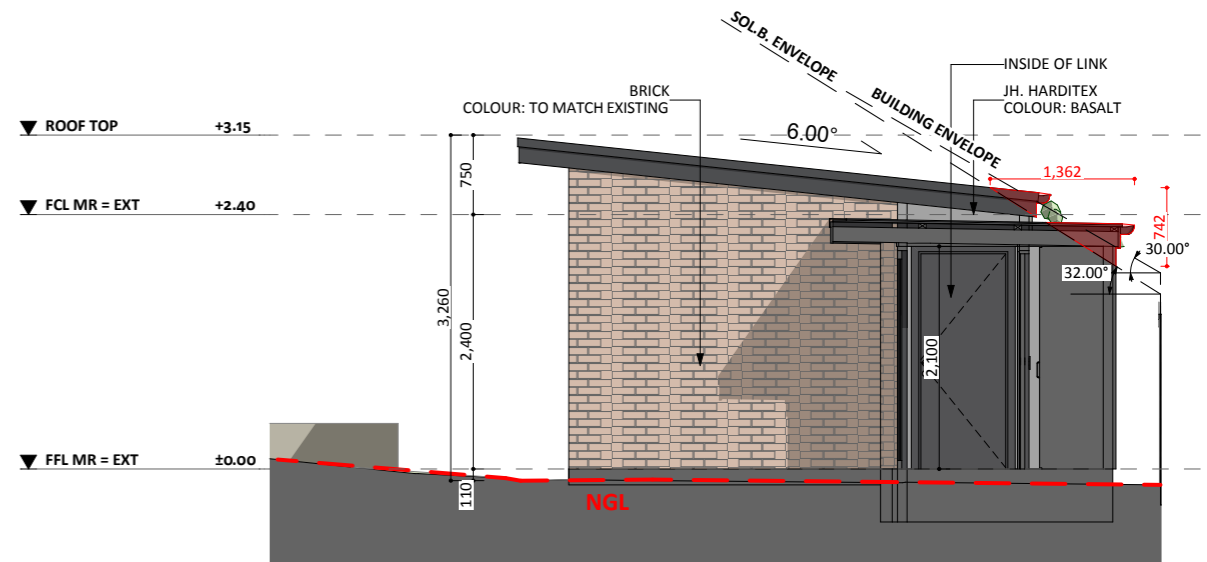
ELEVATION 04
