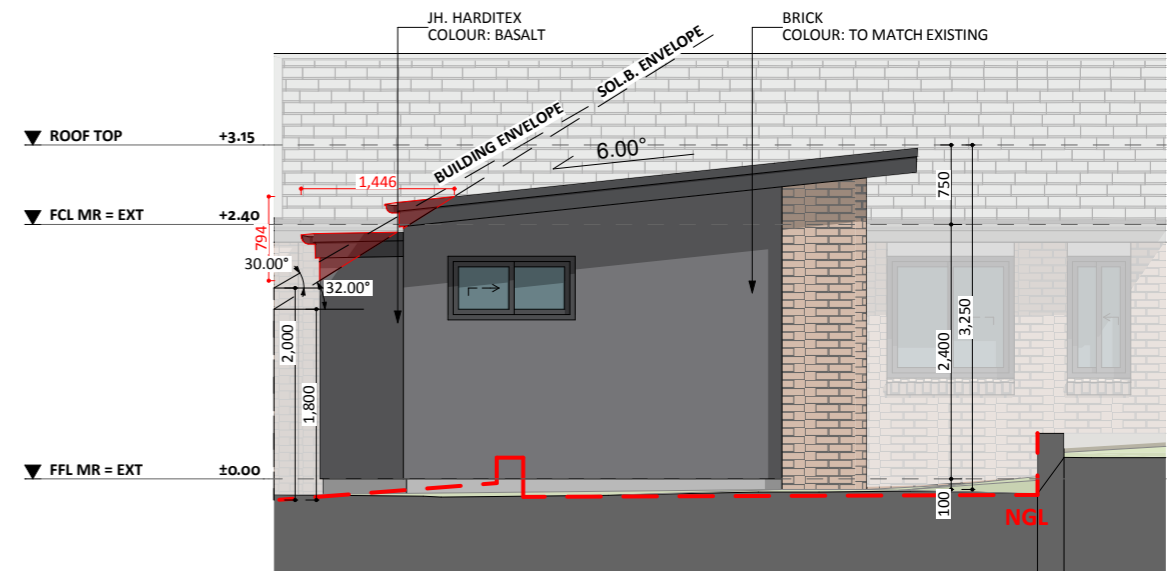
ELEVATION 02
