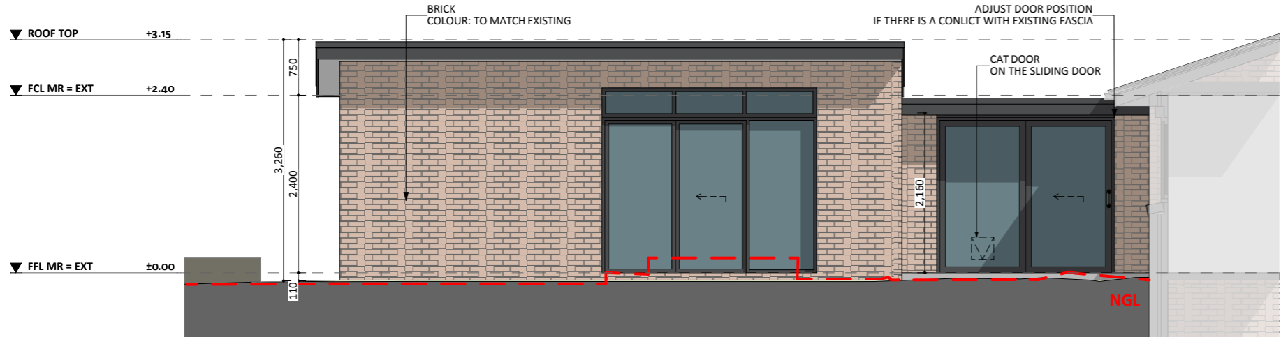
ELEVATION 01
