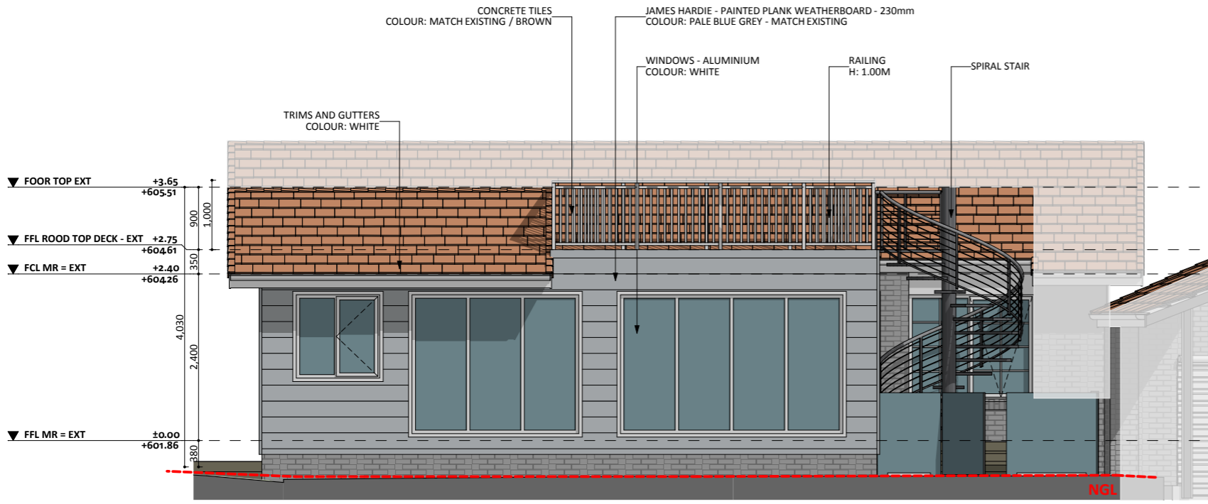
ELEVATION 01
