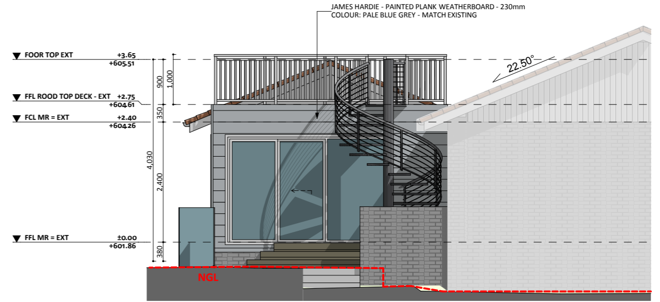
ELEVATION 02
