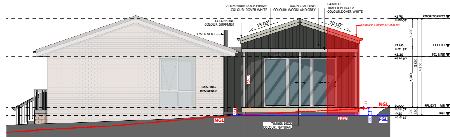
ELEVATION 01
