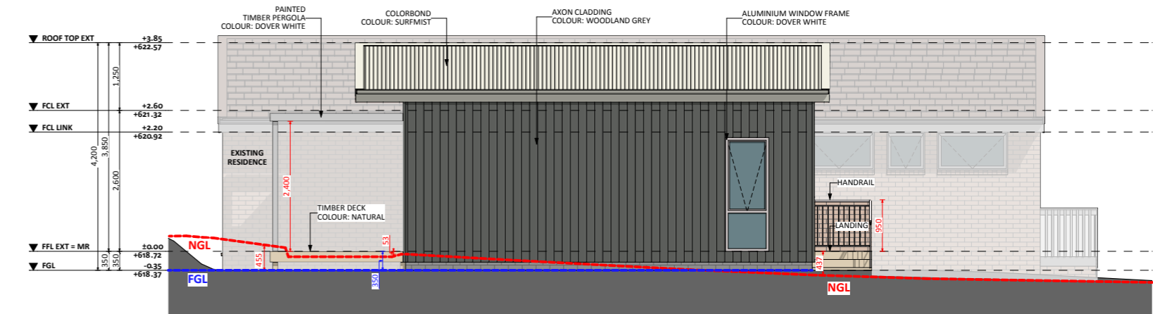
ELEVATION 02
