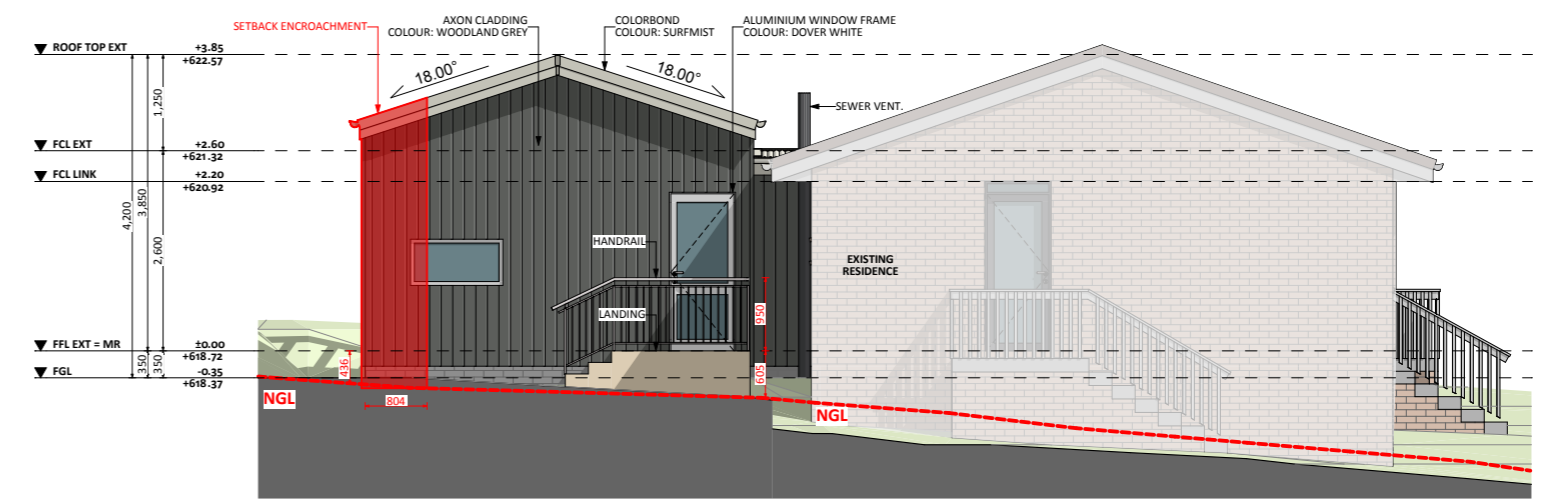
ELEVATION 04
