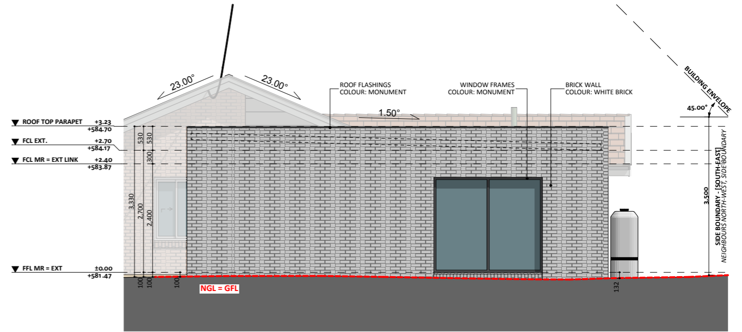
ELEVATION 02
