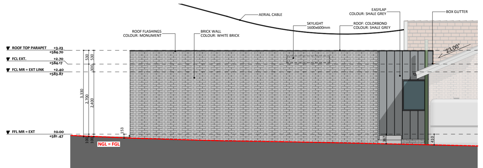
ELEVATION 04
